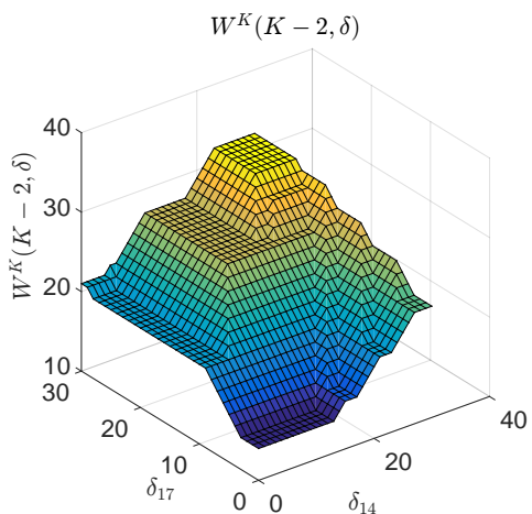
Fig. 7. W^K(K, \delta) .
