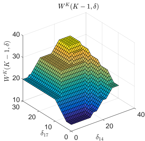
Fig. 6. W^K(K-1, \delta) .
