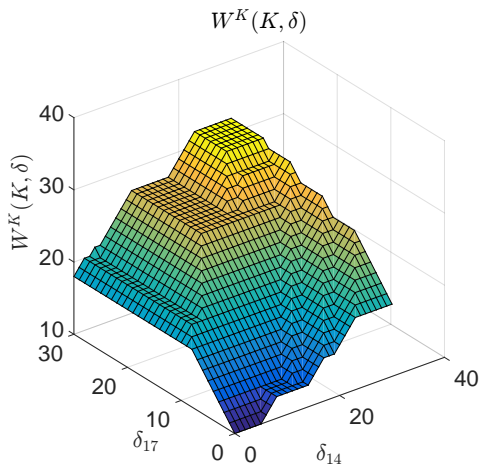
Fig. 5. W^K(K, \delta) .
